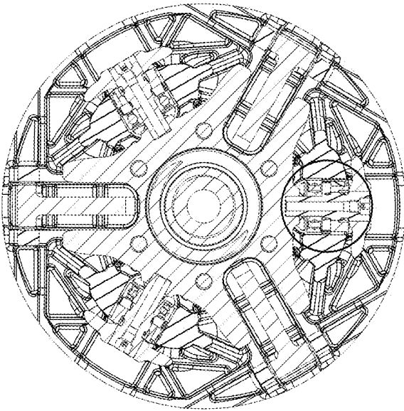
SECTION D-D
