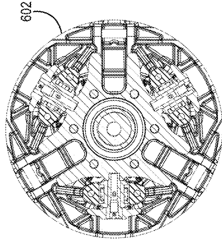
SECTION B-B FIG. 23F
