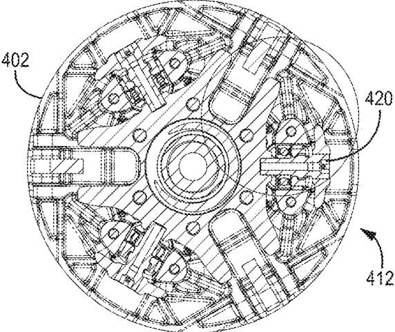
SECTION B-B FIG. 6G
